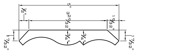
# 17 CROWN -C-5"
